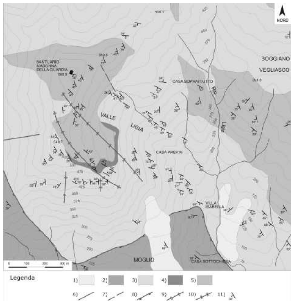
Fig. 2 - Carta geologica dell'area interessata dalla "frana della Liggia" (da Marini, 1989; modificato e ridisegnato). Non è stato riportato l'accumulo di frana. Legenda: 1) coltri detritiche (spessore >3 m); 2) Peliti di Moglio; 3) Calcari di Ubaga; 4) conglomerati mediani e basali; 5) Quarziti di M. Bignone; 6) faglie; 7) faglie presunte; 8) contatti tettonici; 9) assi di pieghe antiformali; 10) assi di pieghe sinformi; 11) giaciture degli strati (polarità indistinta).
